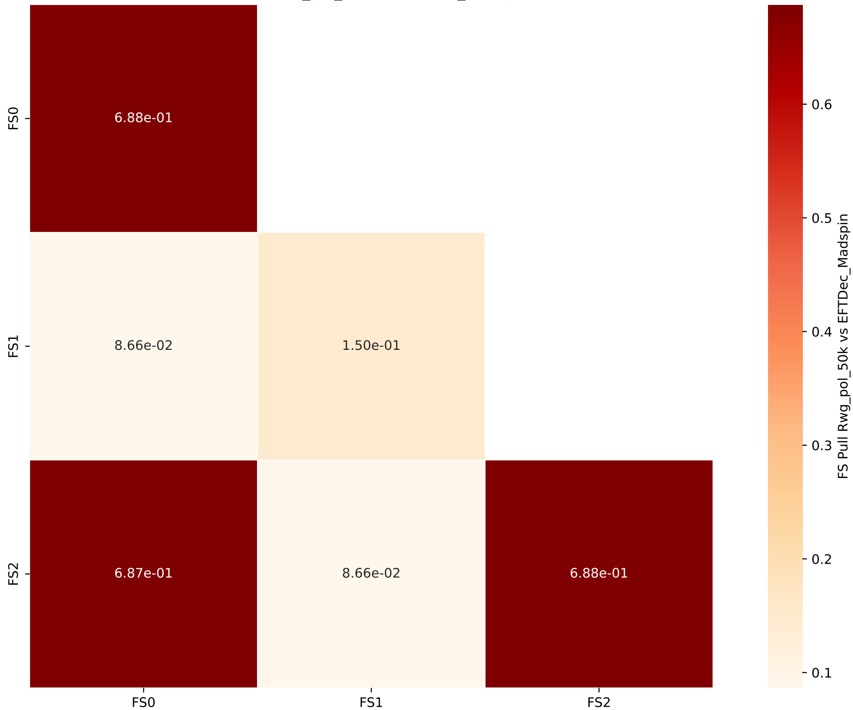
FS Pull Rwg_pol_50k vs EFTDec_Madspin
